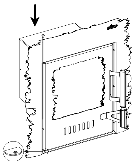
Halterungen
